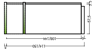
COLONNE H 114 - 150
