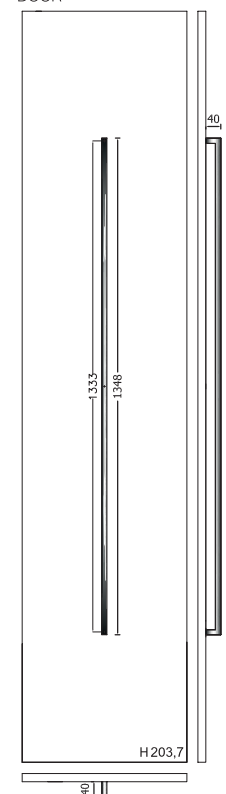
ANTA CESTELLO ESTRAIBILE ESTRAIBILE PULL-OUT BASKET DRAWER DOOR
